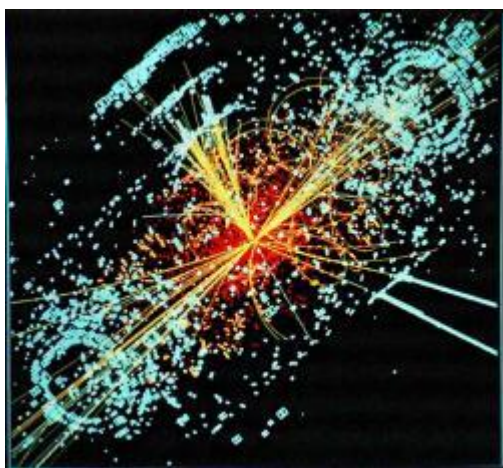
Detekce higgsova bosonu experimentem CMS. Zatím pouze v simulaci. (Zdroj CERN).
