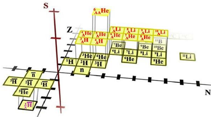
Tabulka dosud nalezených antijader (černé vlevo s horním proužkem) a zatím jediného antihyperjádra (fialové s proužkem), lehkých jader (černé vpravo) a hyperjader (červené vpravo). Na ose x je počet neutronů (N – neutronové číslo), na ose y počet protonů (Z – protonové číslo) a na ose z je počet hyperonů lambda (S – podivnost). (Zdroj BNL)
